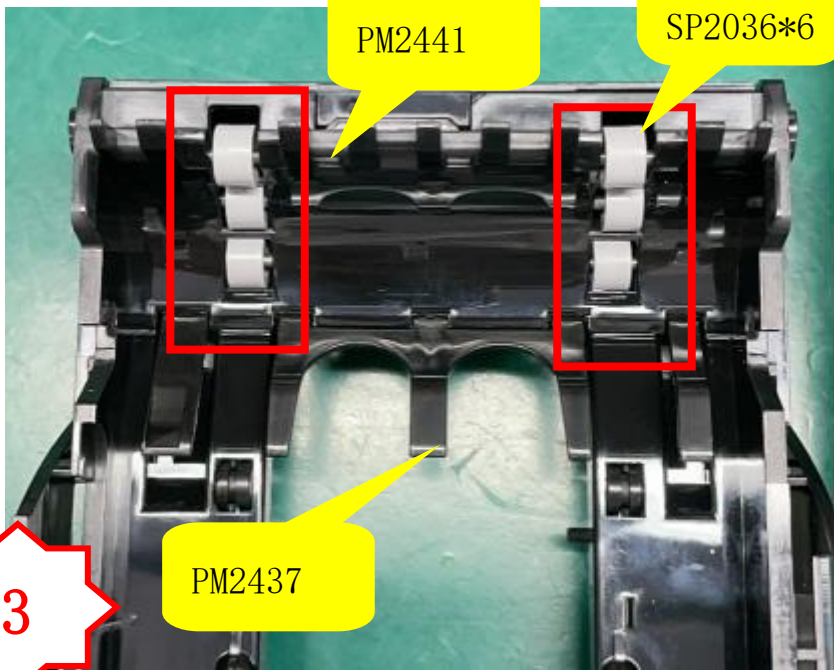
图三, 检查 PM2439, PM2441 是否装配到位, PM2437 是否回弹顺畅
