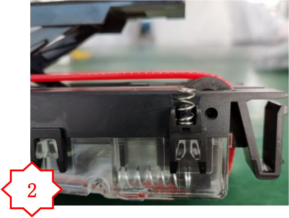
图二，检查 SP125 是否到底无松脱
