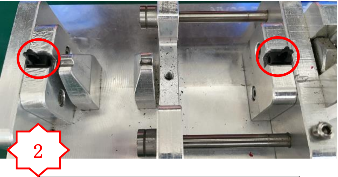
图二，将 2 个 PM2448 装到治具上
