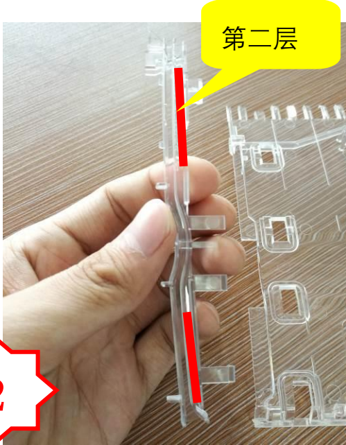
图二，注意用 PM2418 的红色标注部分插入到 PM2415 中
