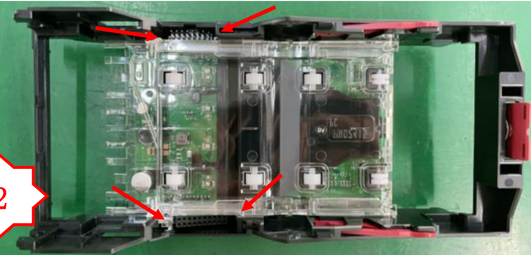
图二，将 PM2415 平放对准连接器用力压进 PM2413 内，注意对应的卡扣压到位，PCBA 板子贴平塑胶件
