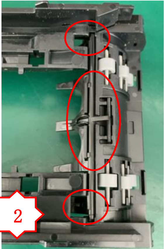
图二，将 PM2437 装配到 PA2612-2 中，检查是否装到位
