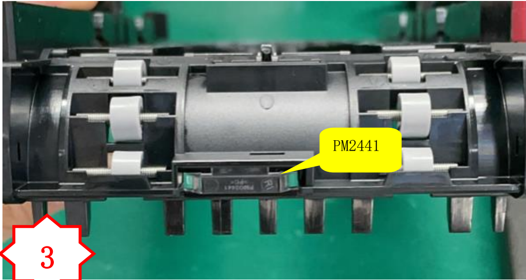
图三，装上一个 PM2441 导光柱
