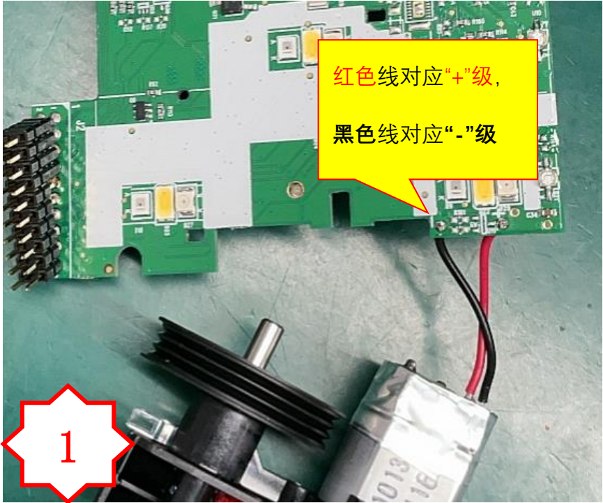
图一，将马达线焊接在 PA2664-1 的正负极，红色对应正级，黑色对应负级。
