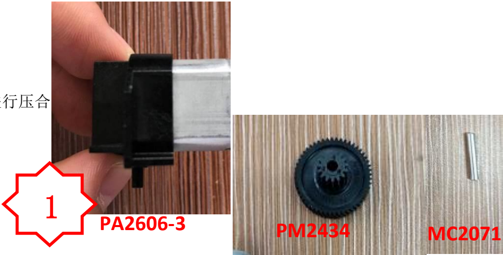
图一, 物料识别
