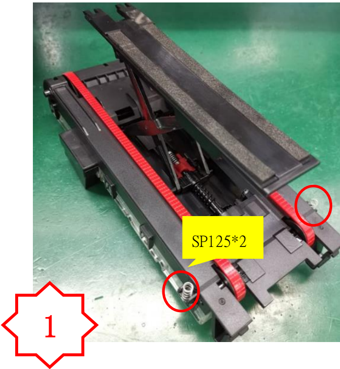
图一，将 2 个 SP125 打到底
