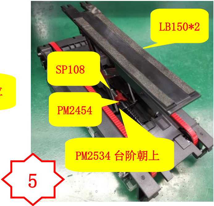
图五, 检查 SP108, PM2454, PM2534, LB150 是否装配到位
