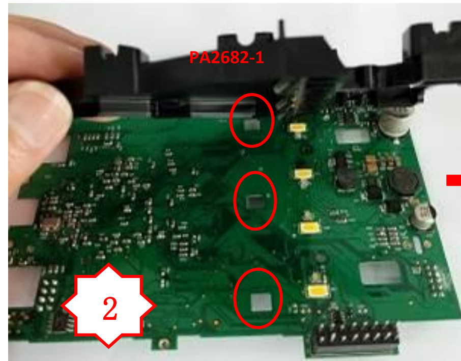
图二, 把 PA2254 和 PA2682-1 装配在一起
