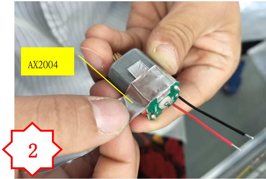
图二，贴上 AX2004，铝箔需沿着马达板边缘，无缝隙
