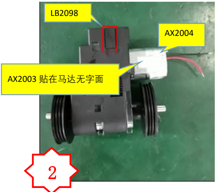
图二，检查铝箔有无漏贴，贴错
