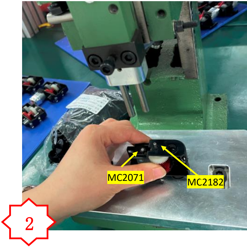
图二，将齿轮箱组件放到治具上，然后放入 MC2071 和 MC2182 将轴压到位
