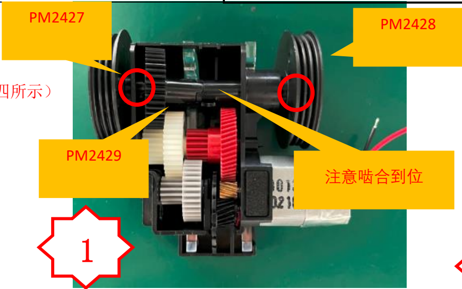
1. 将 3 个齿轮如图放置, 注意啮合到位
