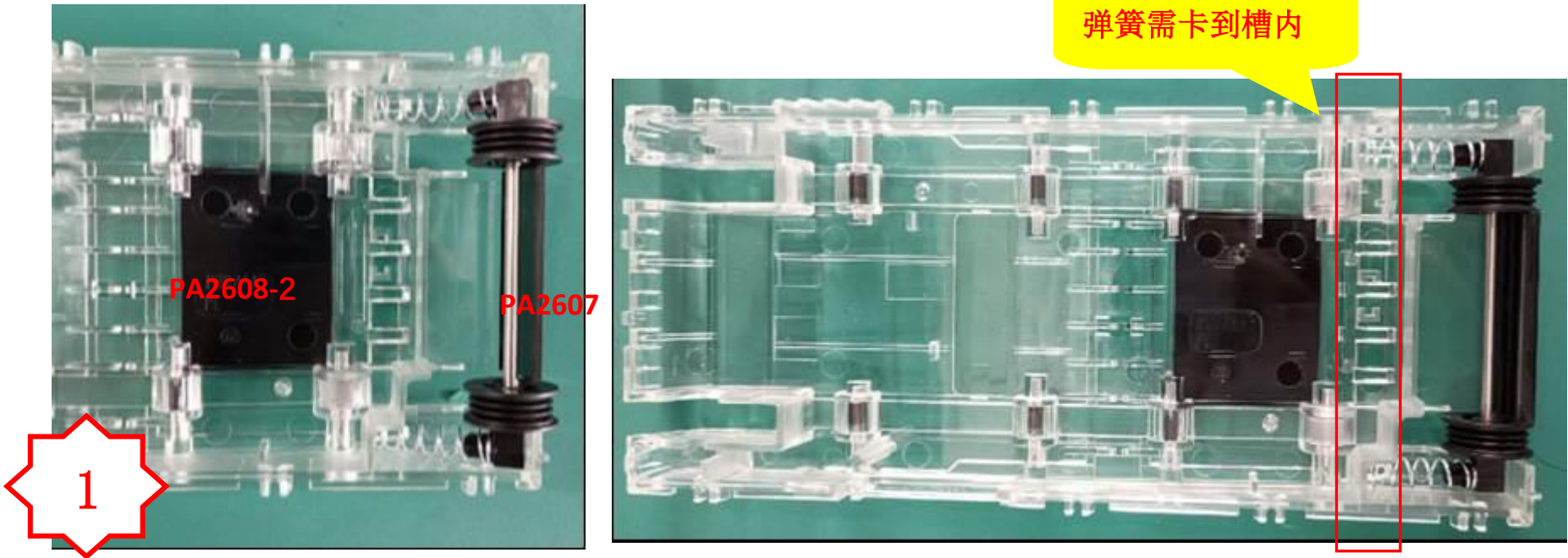
图一, 将 PA2607 装入 PA2608-2
