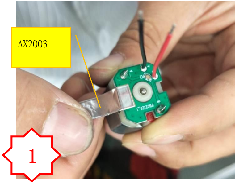
图一，贴上 AX2003，铝箔需覆盖马达板铜片
