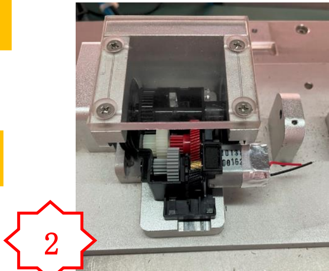
2. 将齿轮箱组件放入治具
