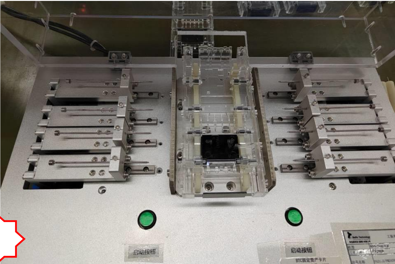
图一，将 8 个 SP2084 用治具压到位
