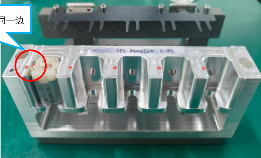
图一, 认真阅读治具提示, 将马达有字一面朝自己放入, 注意马达红点位置与治具上红点位置在同一边
