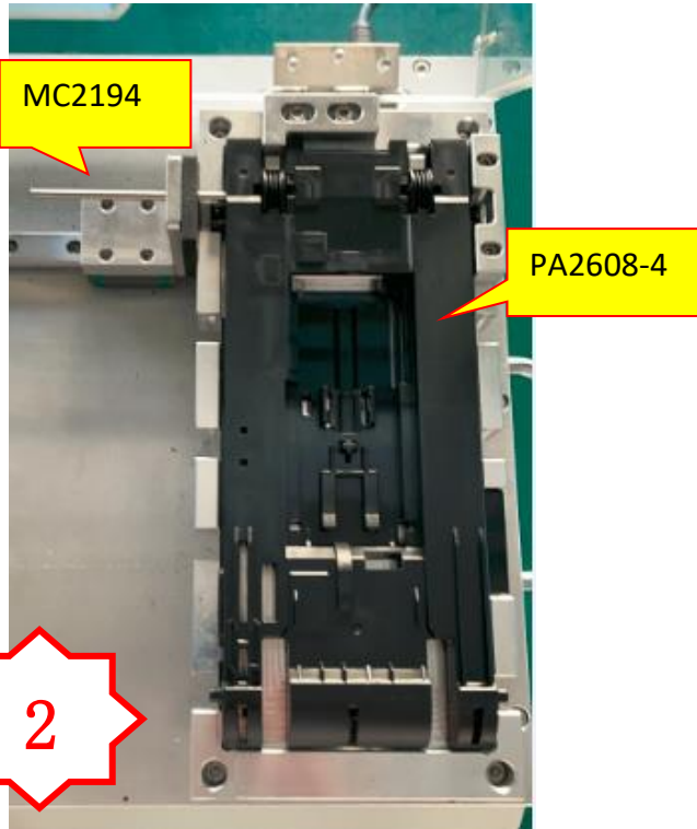
图二, 先将 PA2608-4 放入治具, 在将 MC2194 穿入治具
