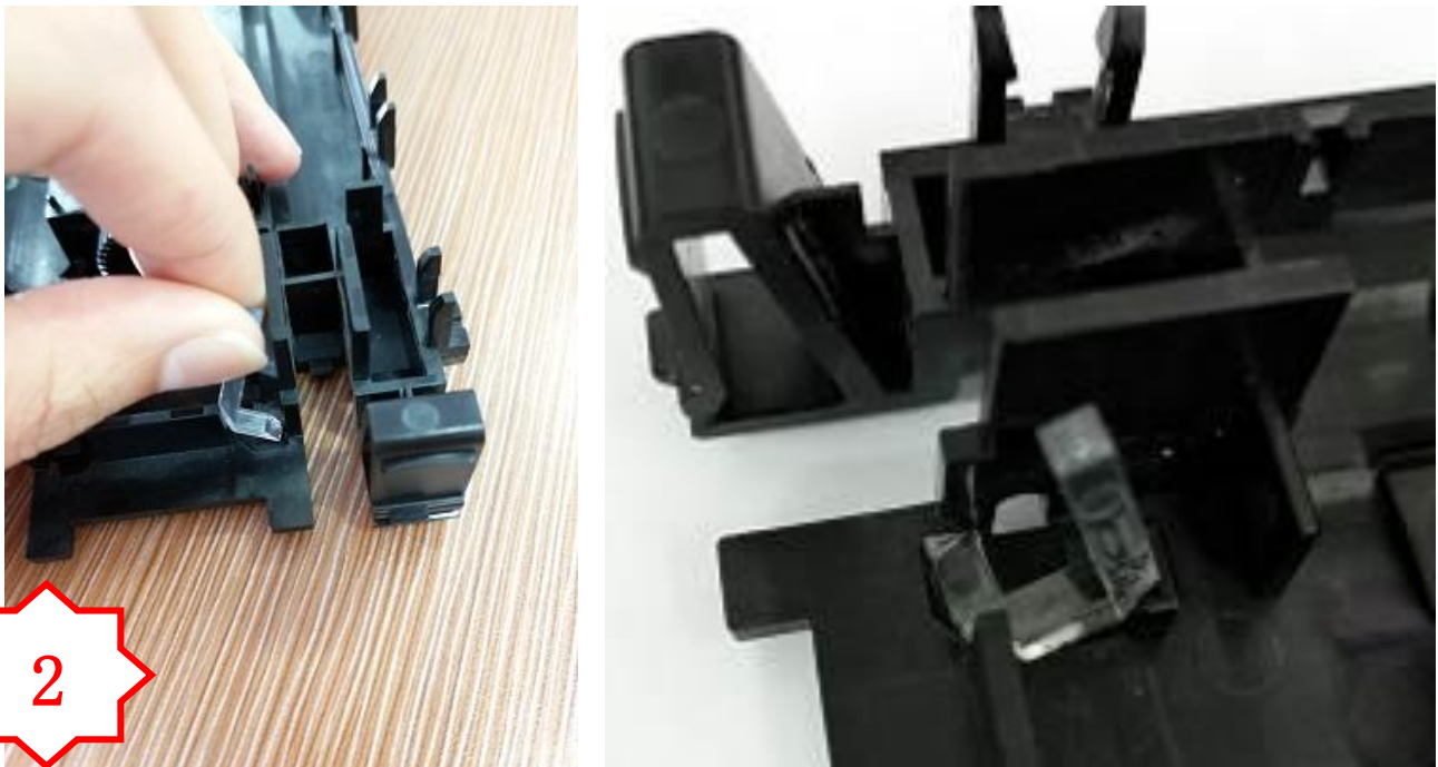
图二，分别将 PM2532 和 PM2533 装入到对应的槽内
