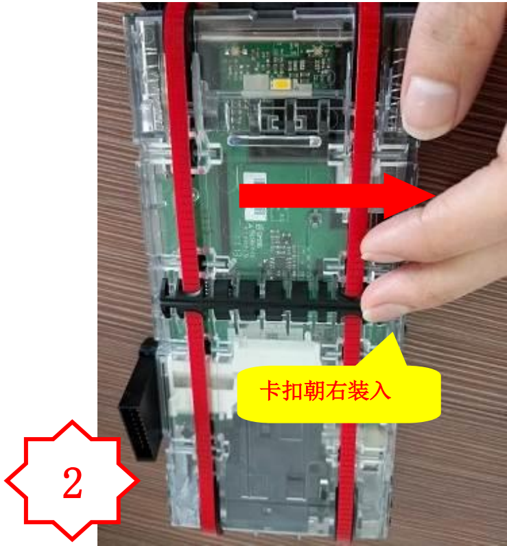
图二, 将 PM2445 装配到 PA2068-9 上
