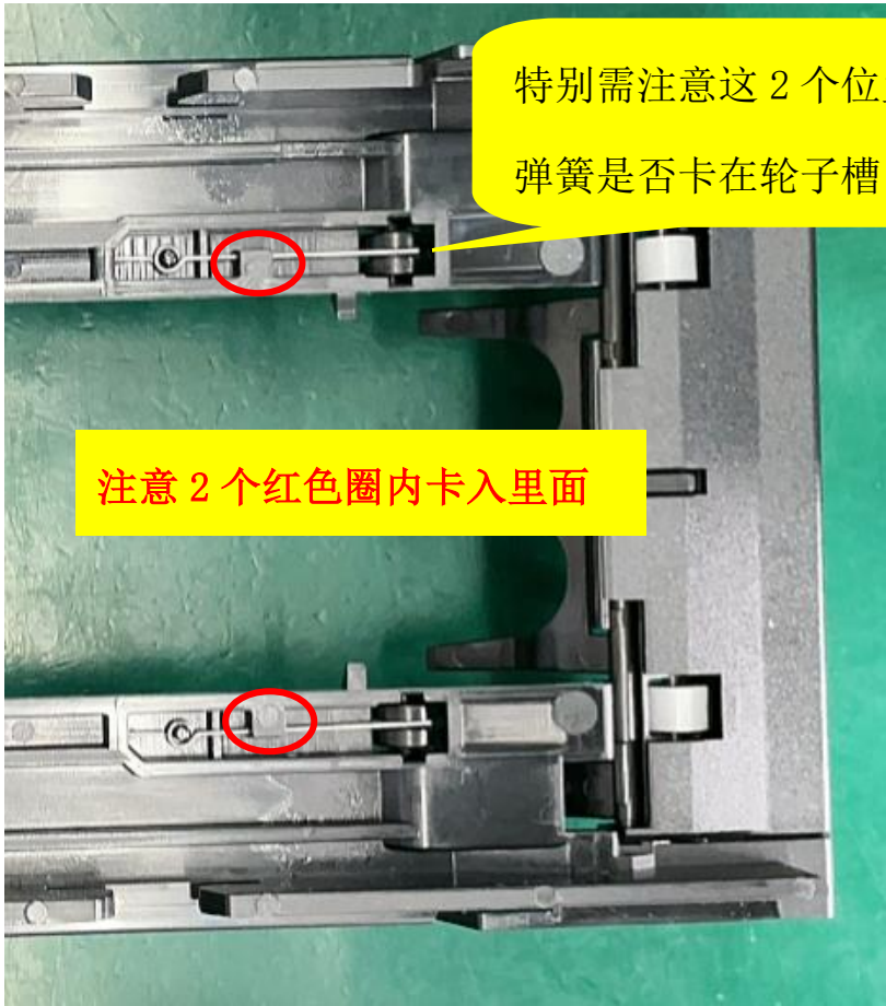
图二，将 PM2440 放入槽中，然后把 SP2034 装配到 PA2612-3 如图所示位置, 共 2 处
