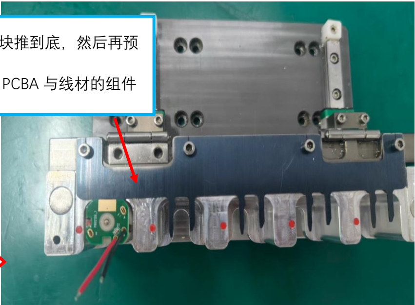
图二, 将治具上的黑色块推向马达, 然后将 PCBA 与线材的组件预装进治具
