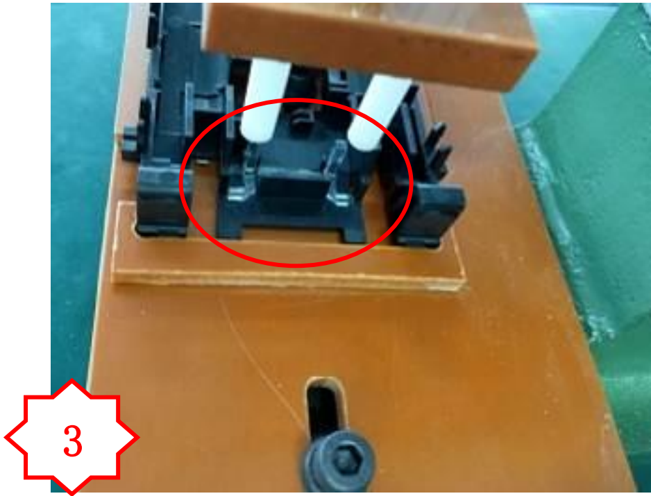
图三，用治具将 PM2532 和 PM2533 压合到位
