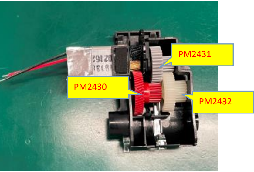
图四, 如图放置齿轮
