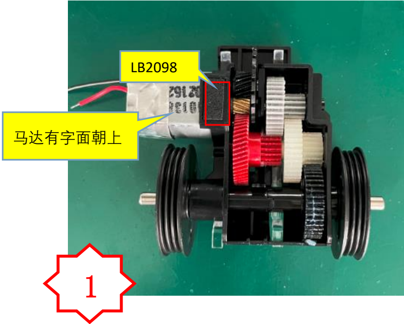
图一，检查齿轮，导光柱，LB2098 有无漏装，马达有字面朝上，齿轮转动是否顺畅
