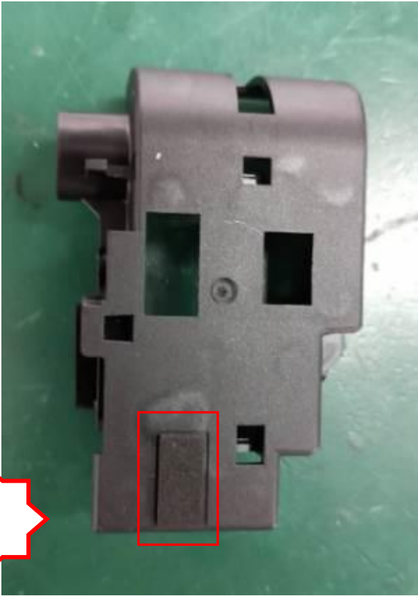
图二, 分别在如图所示两个位置贴上一个 LB2098
