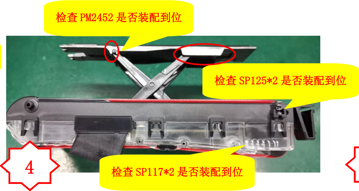
图四, 检查 PM2452, SP117, SP125 是否装配到位
