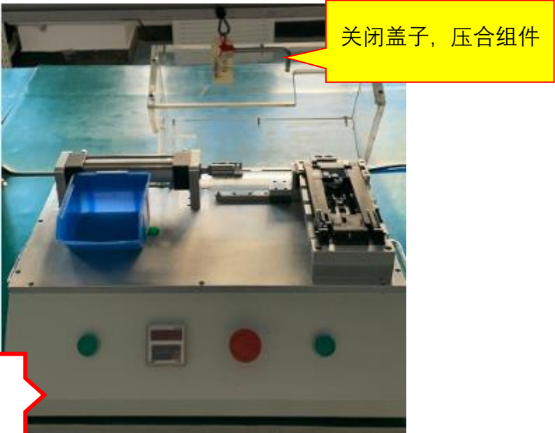
图三, 关闭盖子压合组件
