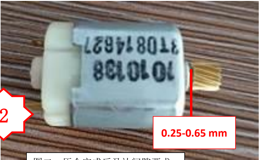
图二，压合完成后马达间隙要求
