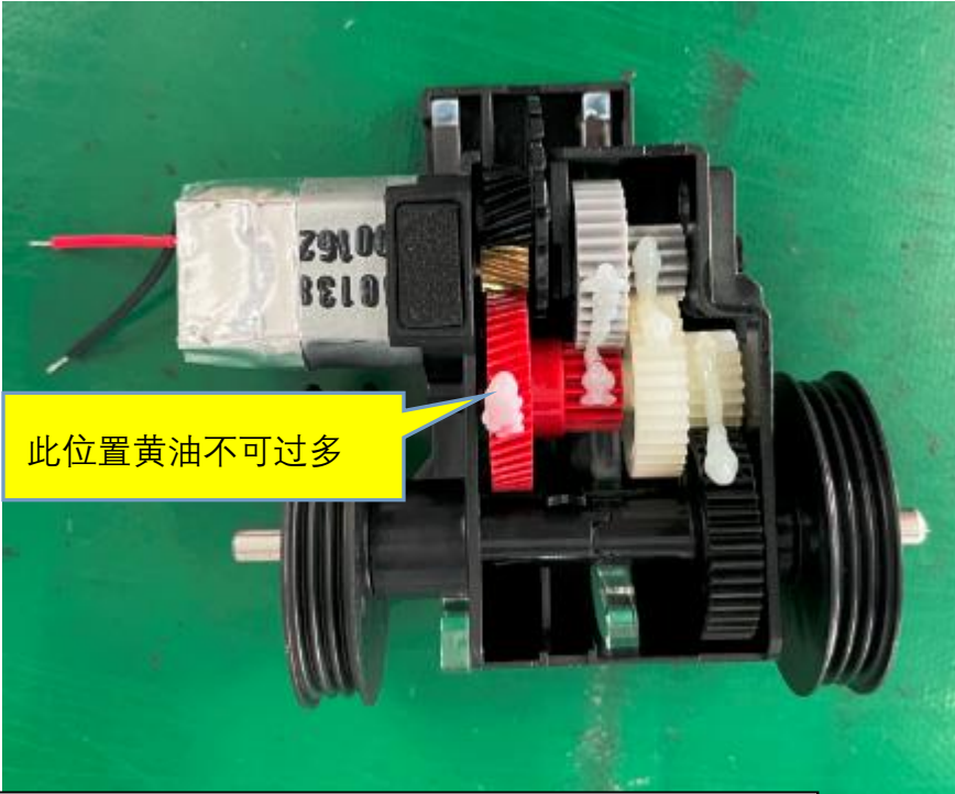
图一，在图中位置点 4 处黄油，用量与图示差不多即可
