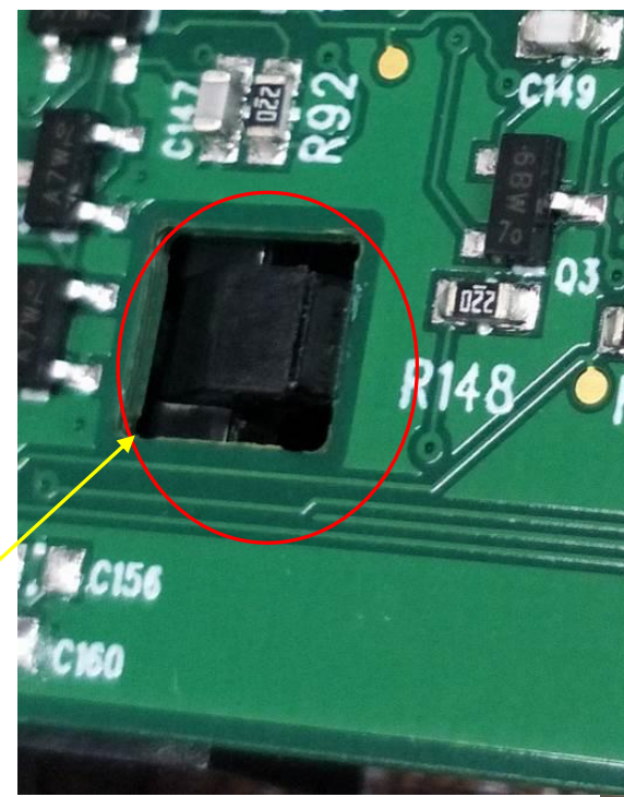
图二, 把 PA2254 和 PA2682-1 装配在一起
