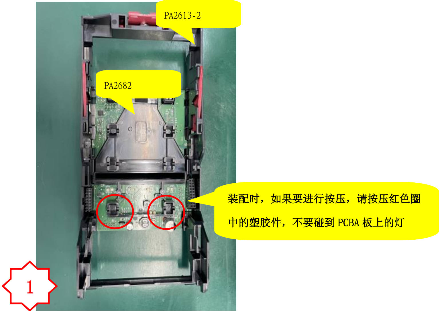
图一, 将 PA2682 放入 PA2613-2 中
