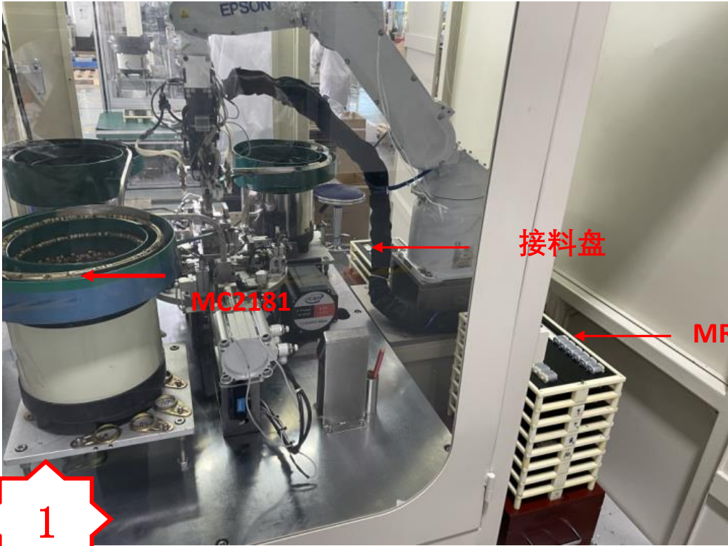
图一，把 MR111 和 MC2181 放到治具中，然后进行压合
