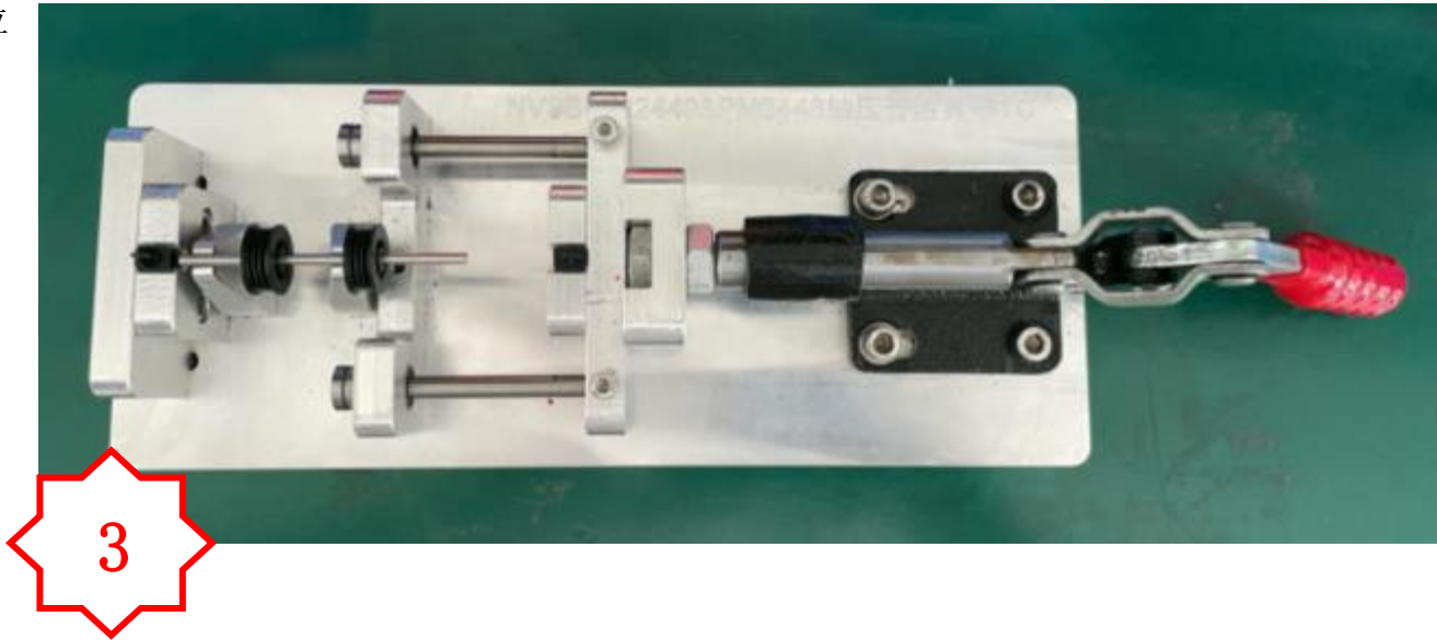
图三，将 2 个 PM2449 穿入 MC2194 后如图放入治具压合
