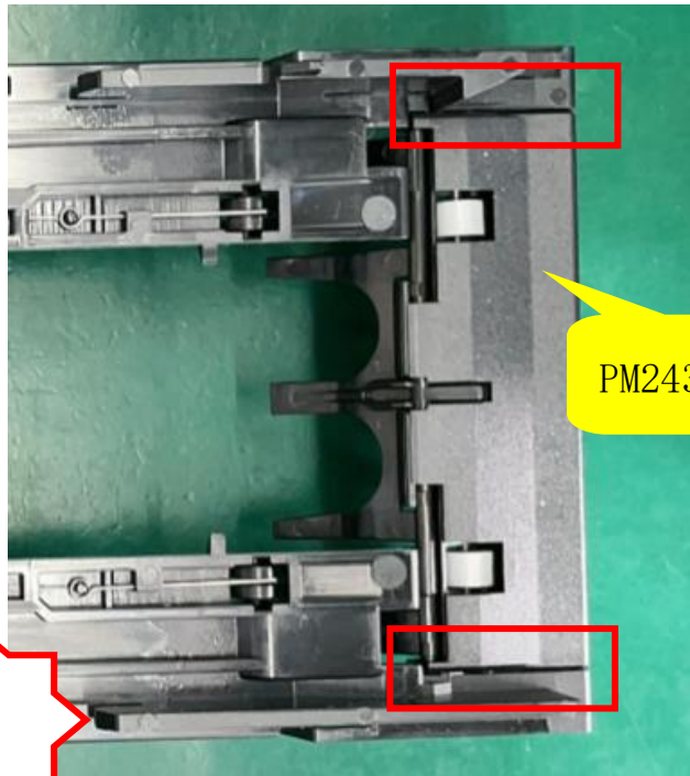
图二, 将 PM2438 装配到 PA2612-2 中, 确保装配后 2 边无突起
