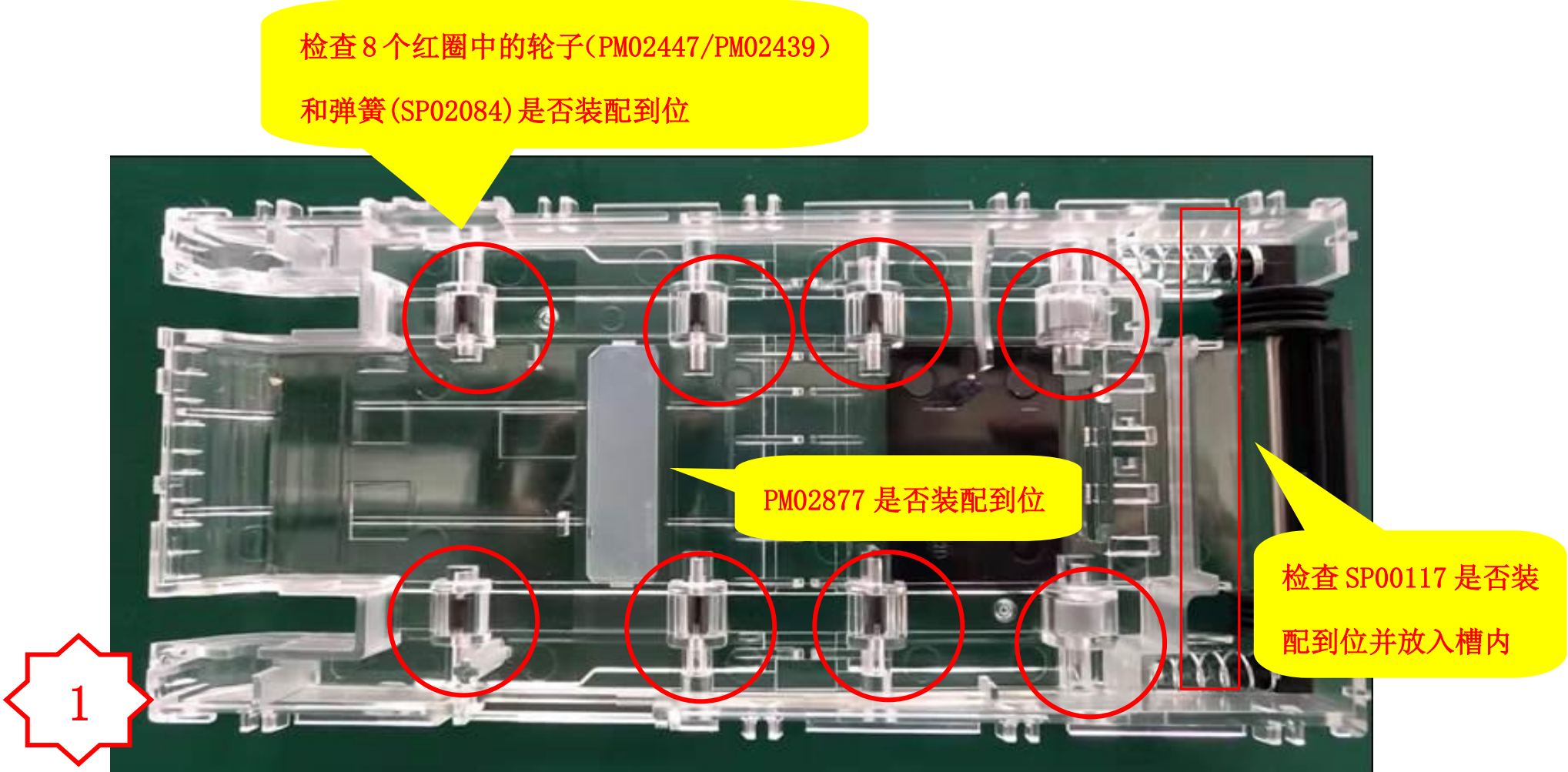
图一，目检图一所示的位置
