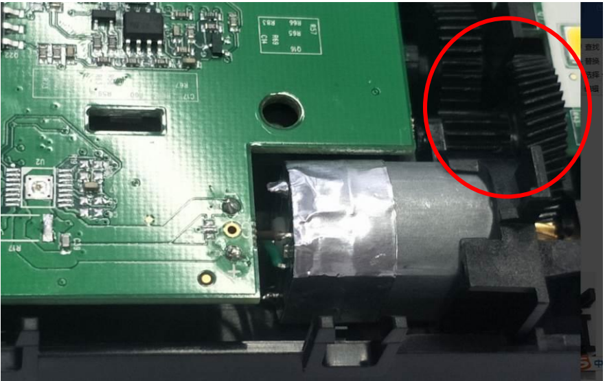
图一，将小马达箱先放入 PA2608-5 的槽位里，齿轮放置到位
