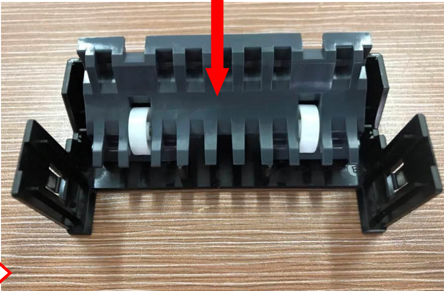
图一, 按照如图所示方向将 PA2792-1 组件卡入到 PM2417 内
