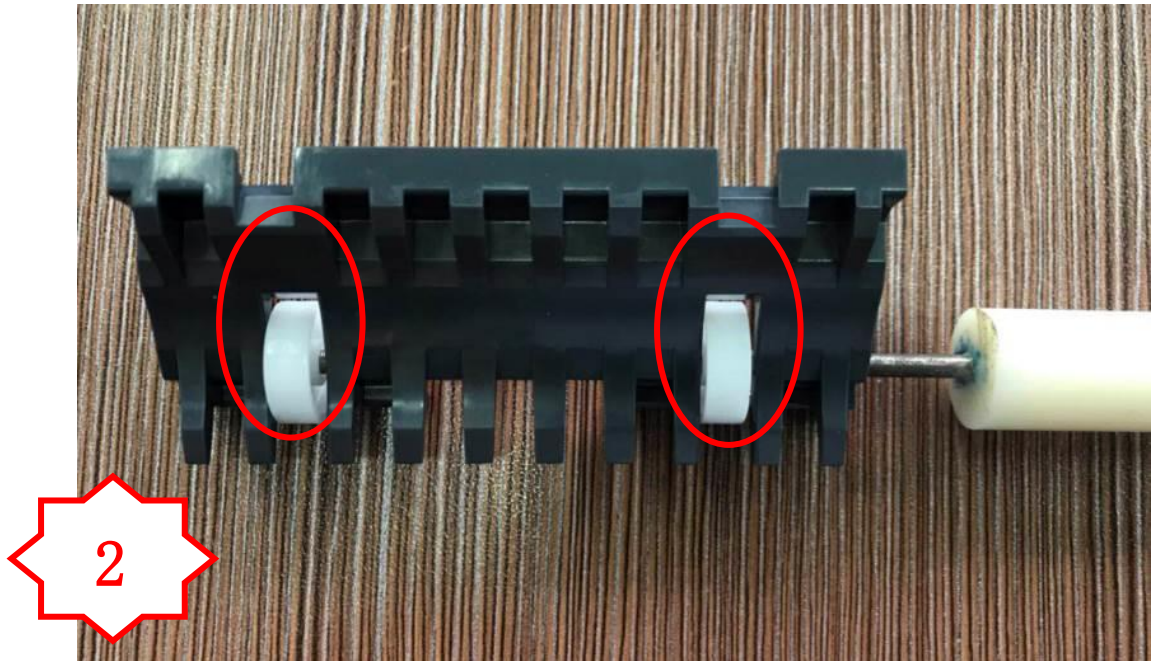
图二，用治具将弹簧压进 PM949 和 PM830 孔内
