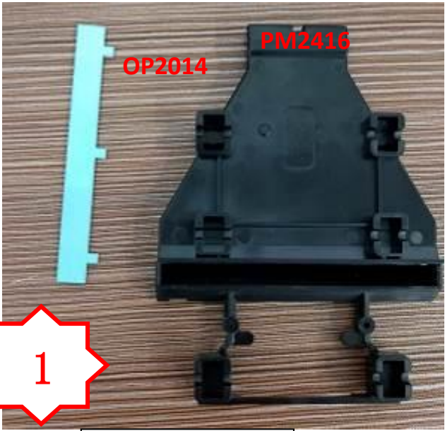
图一, 物料识别
