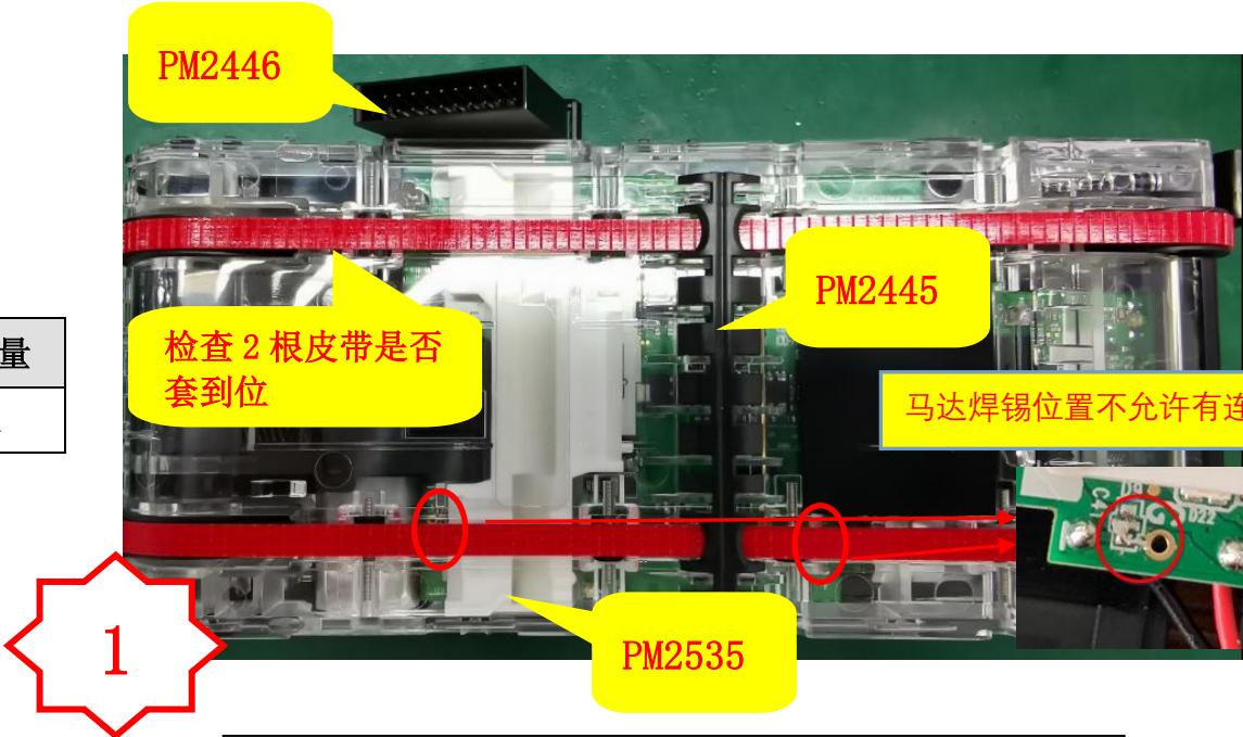
图一, 检查图中标注位置是否装配 OK
