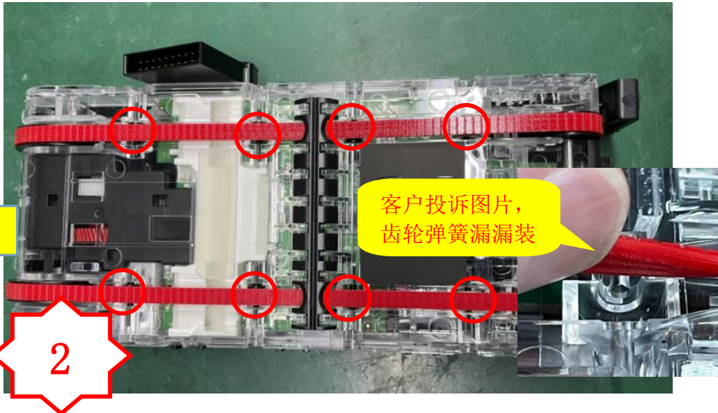
图二, 检查 8 个齿轮及弹簧有无漏装
