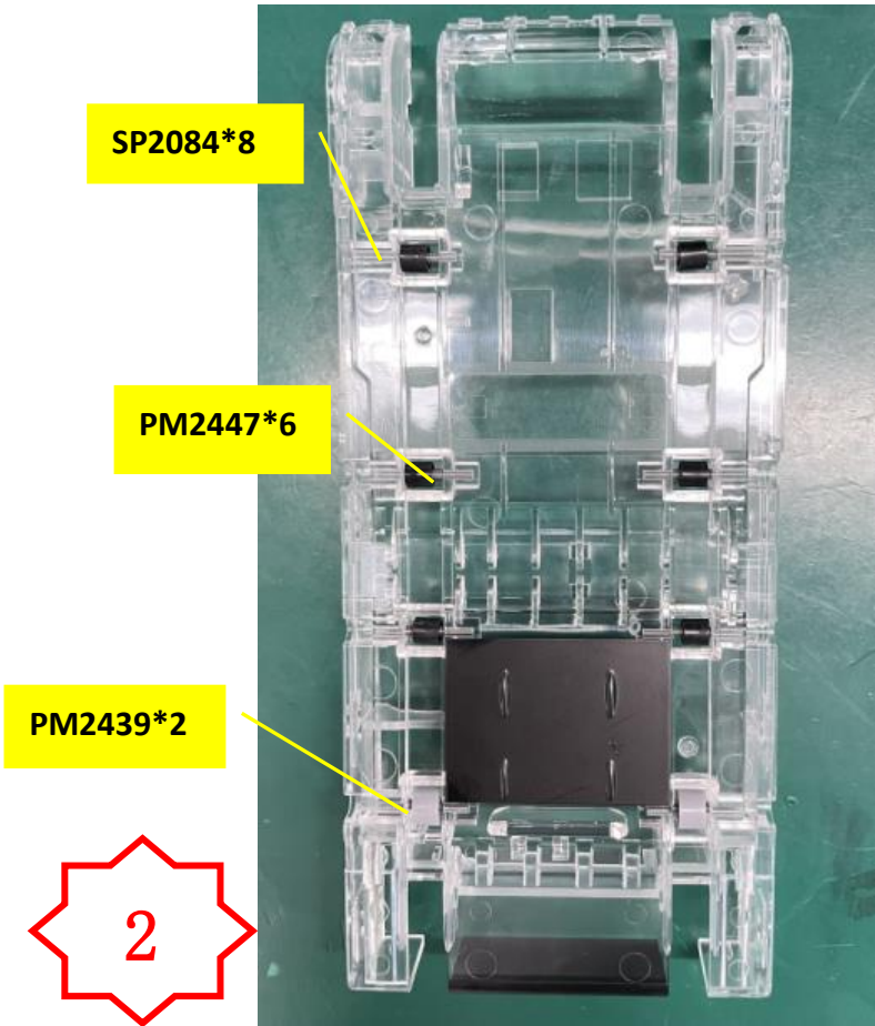
图二，如图在对应位置装上 6 个 PM2447 和 2 个 PM2439, 8 个 SP2084
