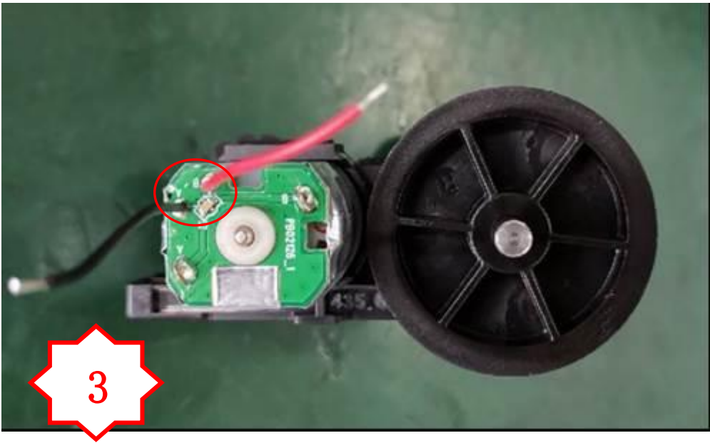
图三，红线在 B 点，黑线在 A 点
