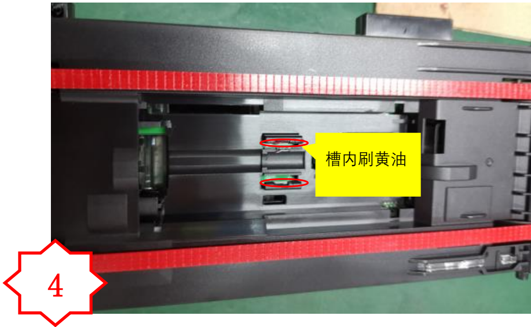
图四, 在图中槽内刷上黄油
