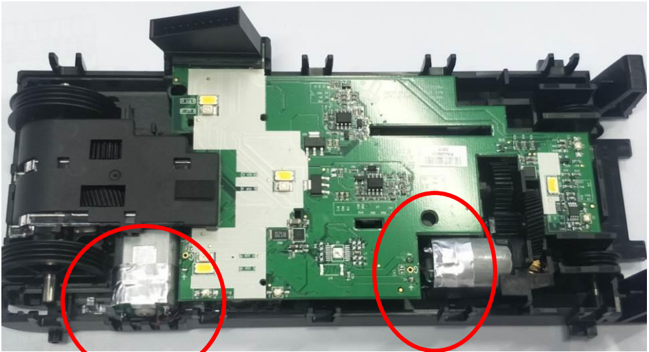
图二，然后将大齿轮箱放置在 PA2608-5 的槽位里，调整好马达线无缠绕，无接触马达本体，PCBA 板。
