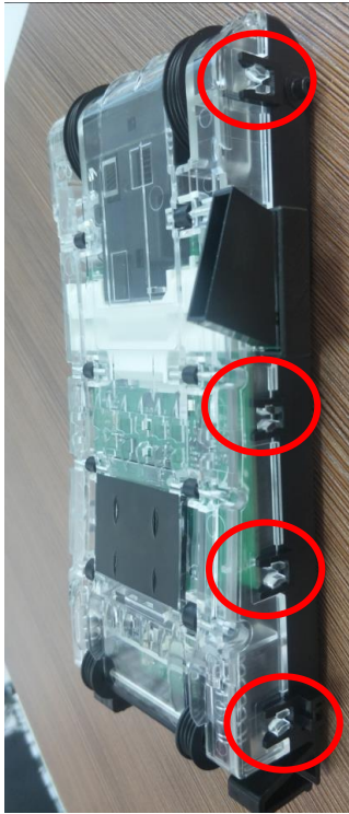
图二, 按图示方向放入组件, 然后双手按 2 个绿色按钮压合, 然后检查 8 个扣位是否到位
