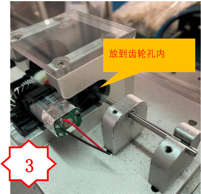
3. 在治具中放入 MC2389
