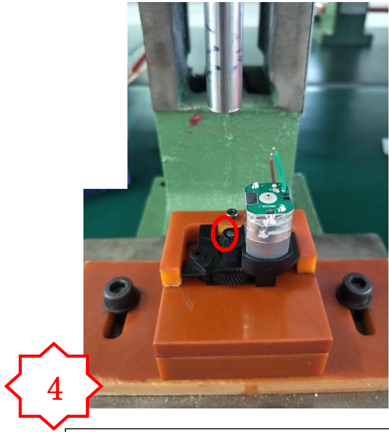
图四, 将装有齿轮的 PA2606-3 放入治具中, 将 MC2071 放到轴孔, 然后进行压合, 压合之后轴的两端与轴孔平齐
