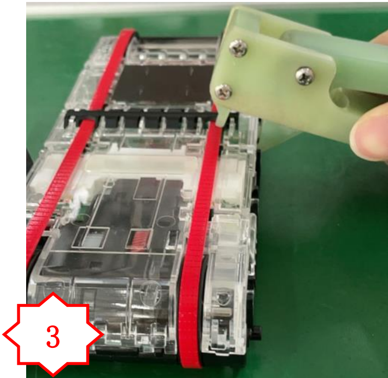
图三, 用自治工具将 PM2445 扣入
