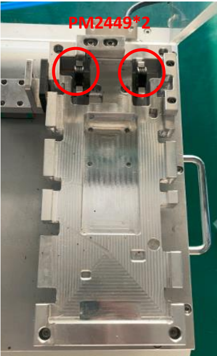
图一, 将 2 个 PM2449 放到红圈的位置
